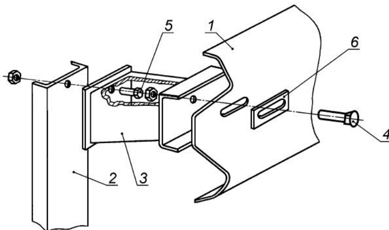
Рисунок А.1 - Одностороннее ограждение дорожной группы с жесткой консолью. Соединение балки со стойкой
