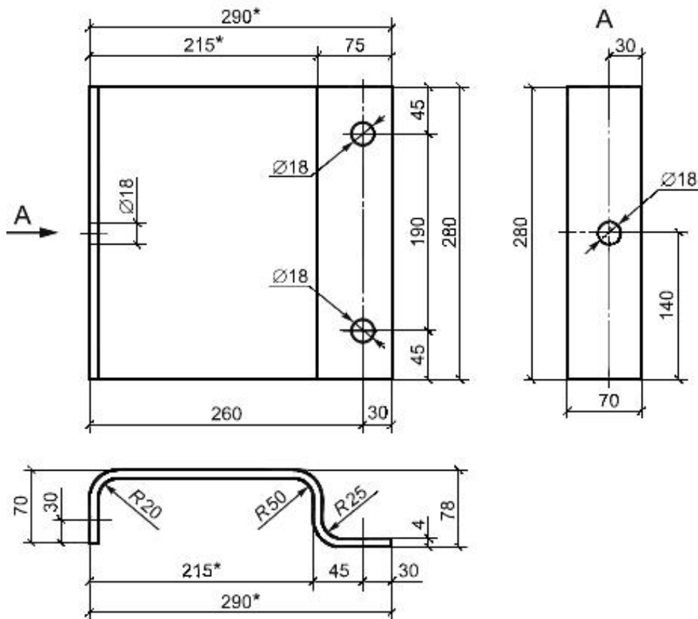
Рисунок 11 - Консоль-амортизатор КА
