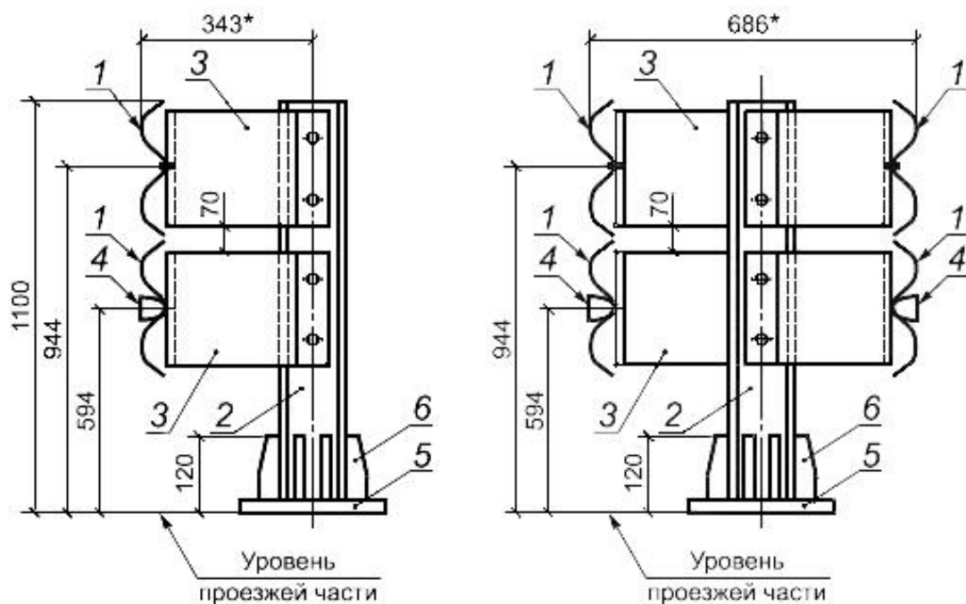
г) Одностороннее двухъярусное ограждение д) Двухстороннее двухъярусное ограждение
