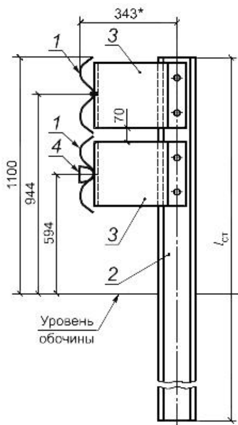
в) Одностороннее двухъярусное ограждение г) Двухстороннее двухъярусное ограждение
