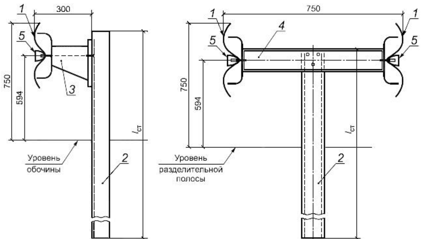
а) Одностороннее ограждение б) Двухстороннее ограждение
